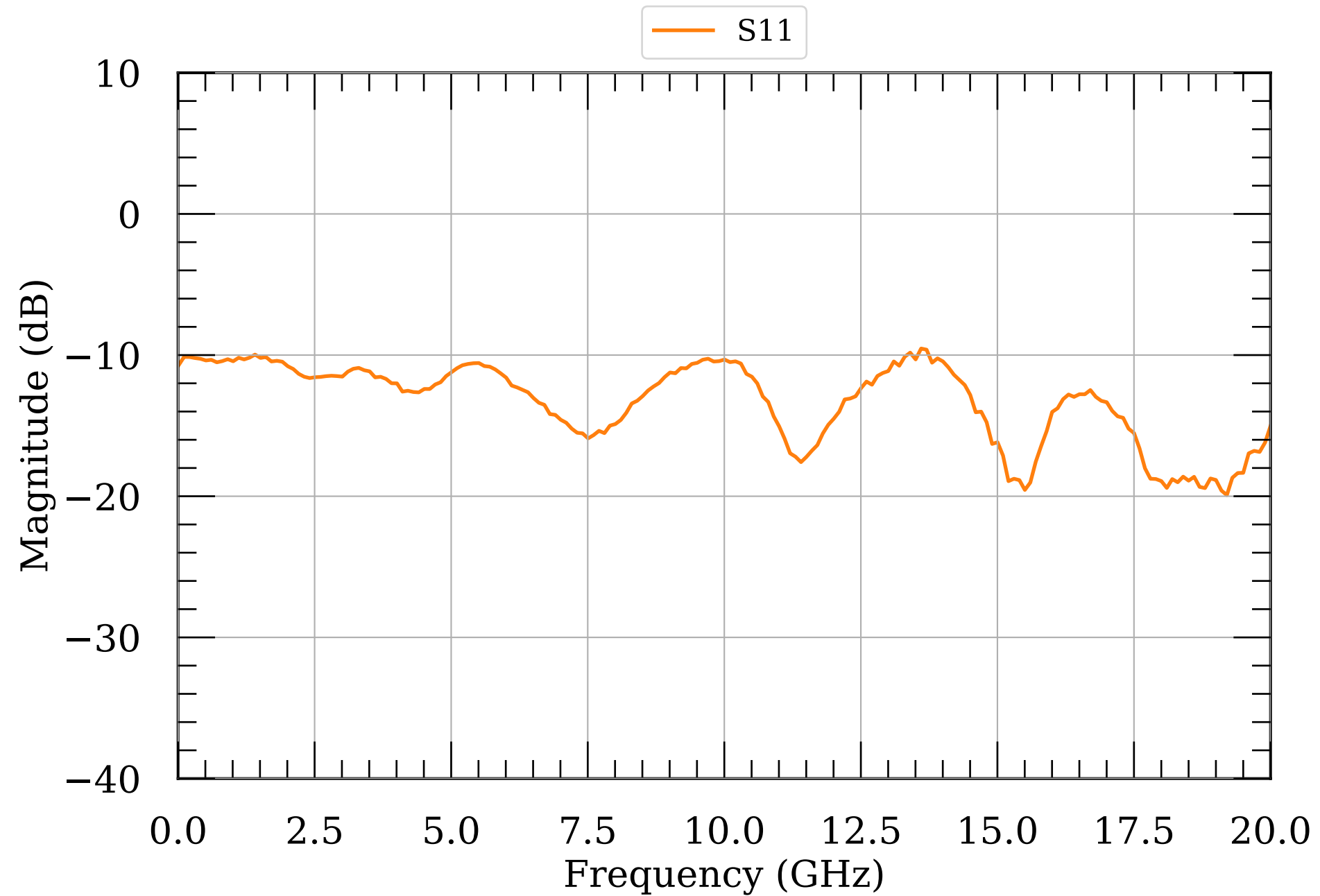
LNA S-params module094v2
